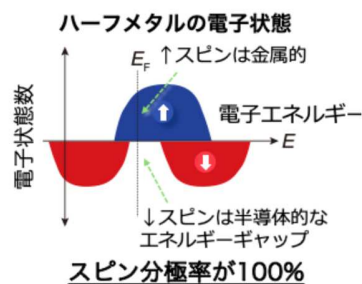
図 1 ハーフメタルの電子状態の模式図
