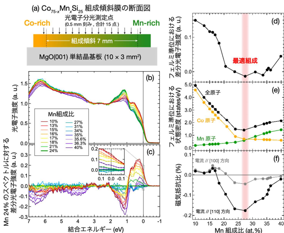
図 3 (a) 作製した Co 75-x Mn x Si 25 組成傾斜膜の構造と光電子分光測定位置、(b)NanoTerasu において測定した価電子帯のスペクトル、(c) Mn 24at.%に対する差分のスペクトル、(d) フェルミ準位(結合エネルギーが 0)上の差分信号の Mn 組成比依存性、(e) (f)フェルミ準位における状態密度の理論計算値と異方性磁気抵抗効果の磁気抵抗比の Mn 組成依存性
